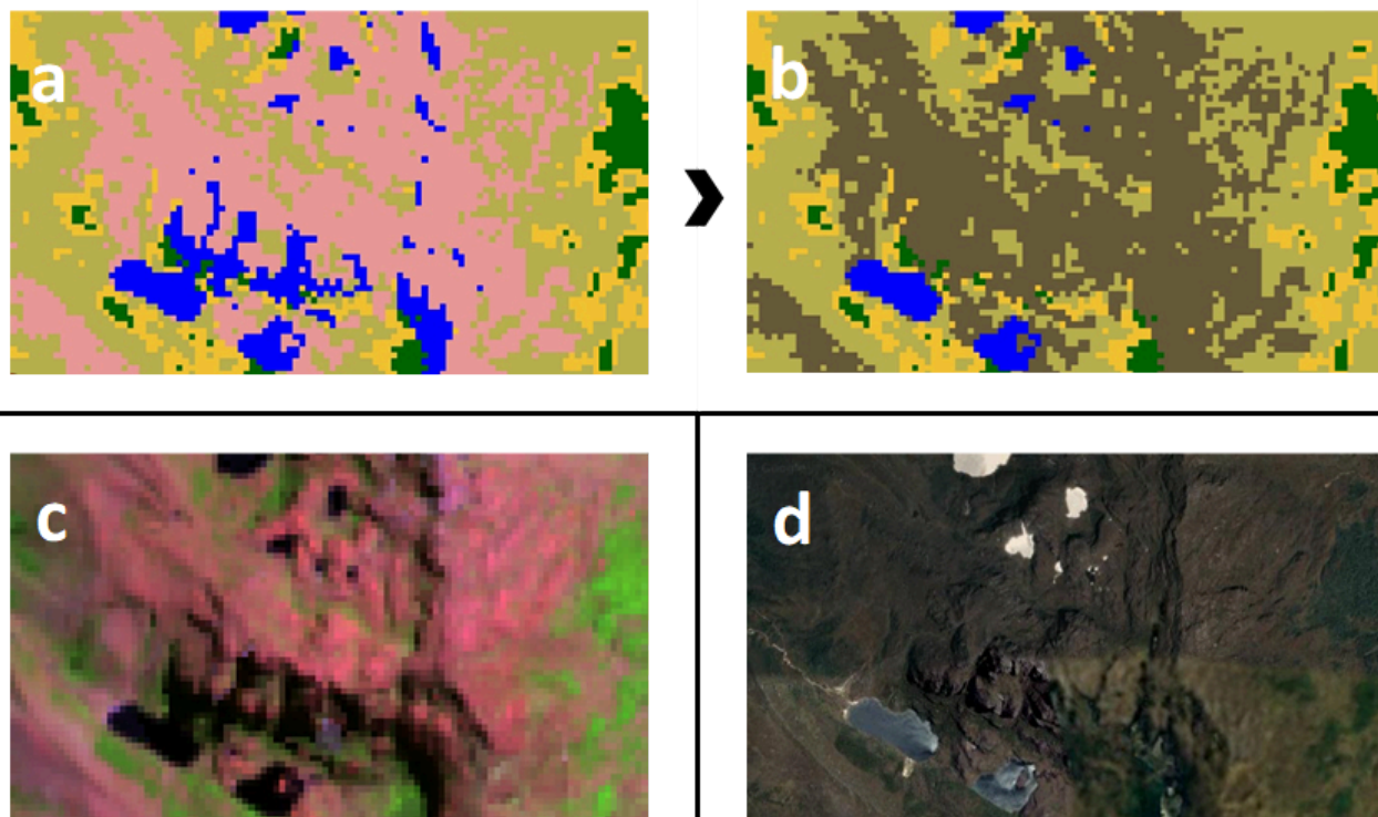
Figura 23. Máscara de afloramiento rocoso (ID 29). a) Clasificación original (antes de la aplicación de la máscara). b) Aplicación de máscara de afloramiento rocoso. c) Mosaico Landsat año 2022 d) Imagen de alta resolución de Google Earth (Elaboración Ecociencia).
