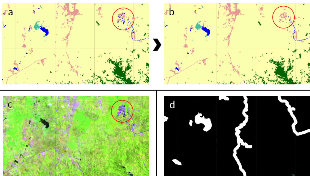
Figura 22. Geometrías de exclusión ( hidden ). a) Clasificación pre filtro. b) Clasificación post filtro de frecuencia. c) Mosaico Landsat año 2022 d) Zona de exclusión en color blanco (Elaboración MapBiomos).
