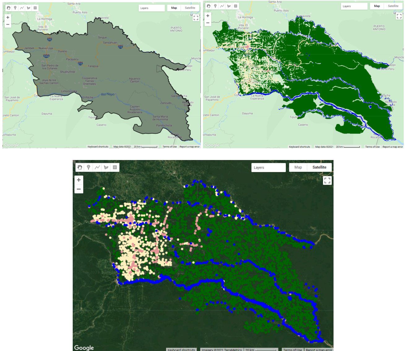
Figura 17. Ejemplo de sorteo de puntos de muestreo de entrenamiento para una región de clasificación de la Amazonía ecuatoriana. a) Límite de la región de clasificación 40201 “Amazonía Baja 1”. b) Mapa de píxeles estables para sorteo de puntos de muestreo. c) Puntos de muestreo sorteados en la región 40201 (Elaboración Ecociencia).
