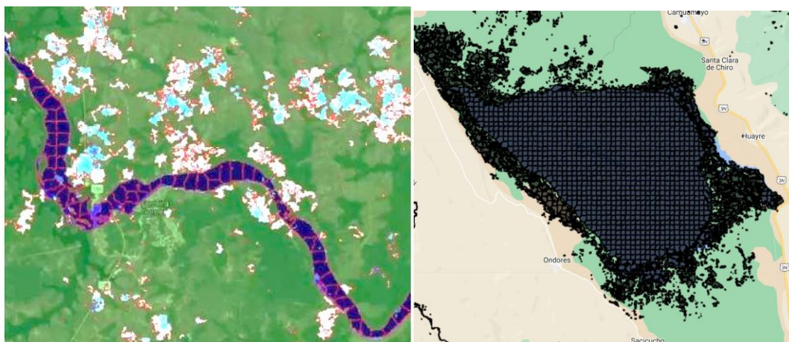
Figura 8. Ejemplos del proceso de segmentación que convierte datos ráster (frecuencia mensual dentro de cada año) en una malla de vectores regulares.
