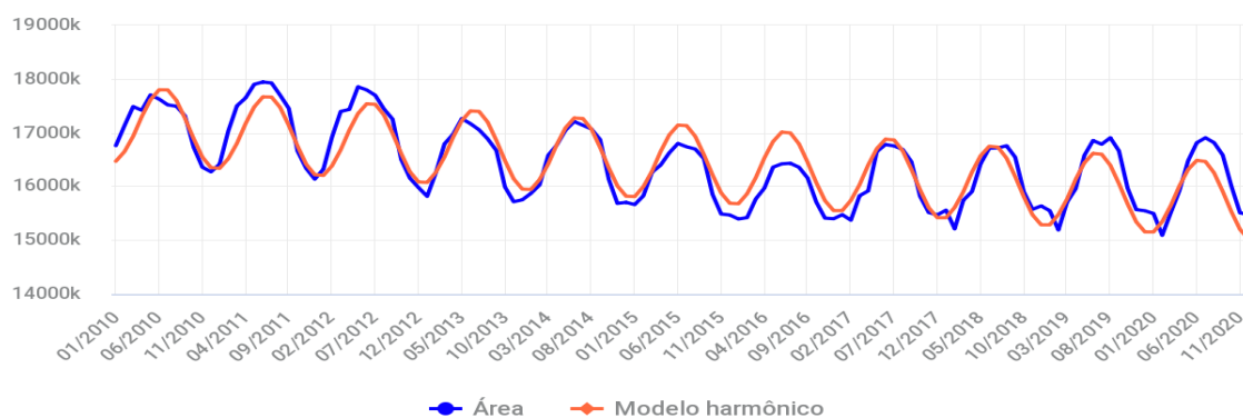
Figura 12. Ejemplo de ajuste de serie armónica a los resultados de superficie de agua mapeada mensualmente. La línea azul corresponde a la superficie de agua mapeada, la línea roja indica el ajuste del modelo armónico.
