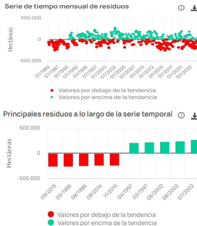
Figura 13. Ejemplo de las diferencias entre el modelo ajustado y los datos observados. Los puntos y barras verdes indican valores de aumento, mientras que los puntos y barras rojas indican valores de disminución en relación con lo esperado por el modelo armónico.
