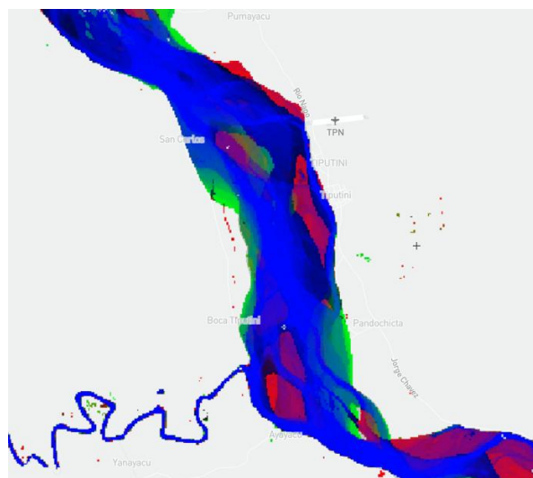
Figura 10. Dinámica de superficie de agua RGB. El color azul indica persistencia, ya que el total de años fueron clasificados como superficie de agua; verde, incrementó (los años desde el principio de la serie temporal hasta la primera clasificación); y rojo disminución. Los colores negros y oscuros indican superficies de agua esporádicas o no permanentes.
