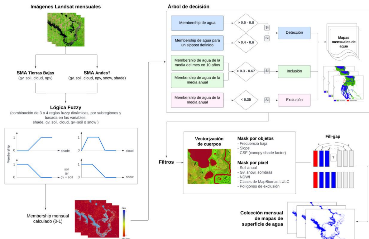
Figura 3. Diagrama del proceso metodológico para producir los datos de superficie de agua, 1985-2025.
