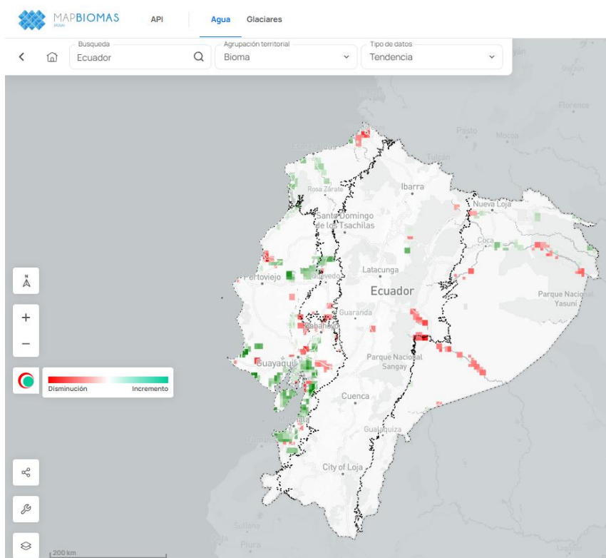
Figura 14. Ejemplo de resultados de cálculo de tendencias para Ecuador utilizando la prueba estacional de Mann Kendall. Los datos en rojo indican una disminución, los datos en verde un aumento y los datos en blanco, estabilidad. Sólo se presentan datos con valores significativos.
